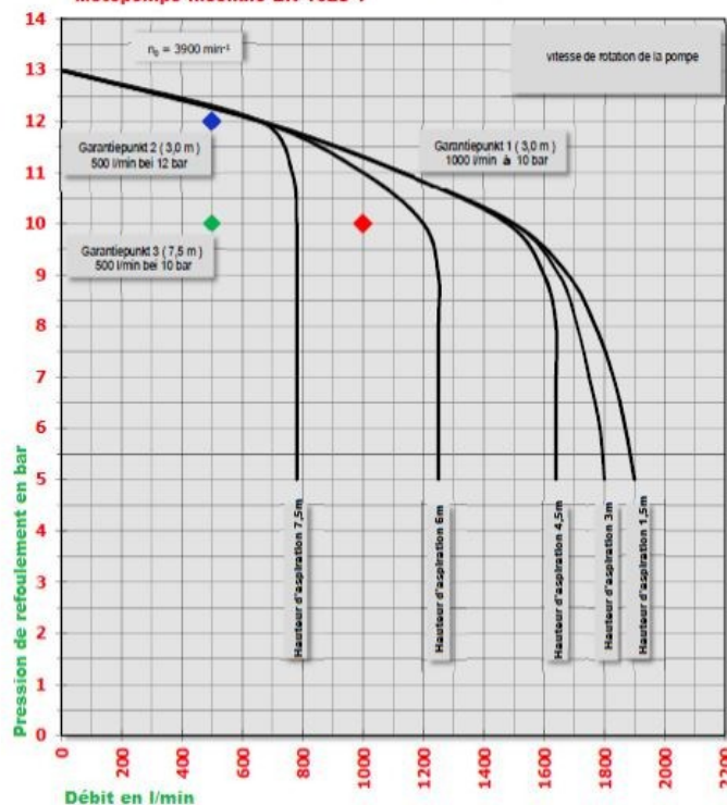
Tests réalisés conformément à la EN 1028-2 Motopompe incendie EN 1028-1
