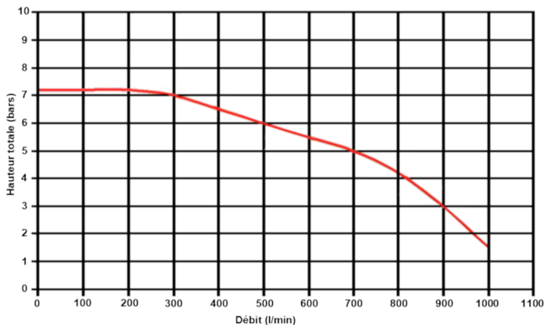
Courbe de puissance
