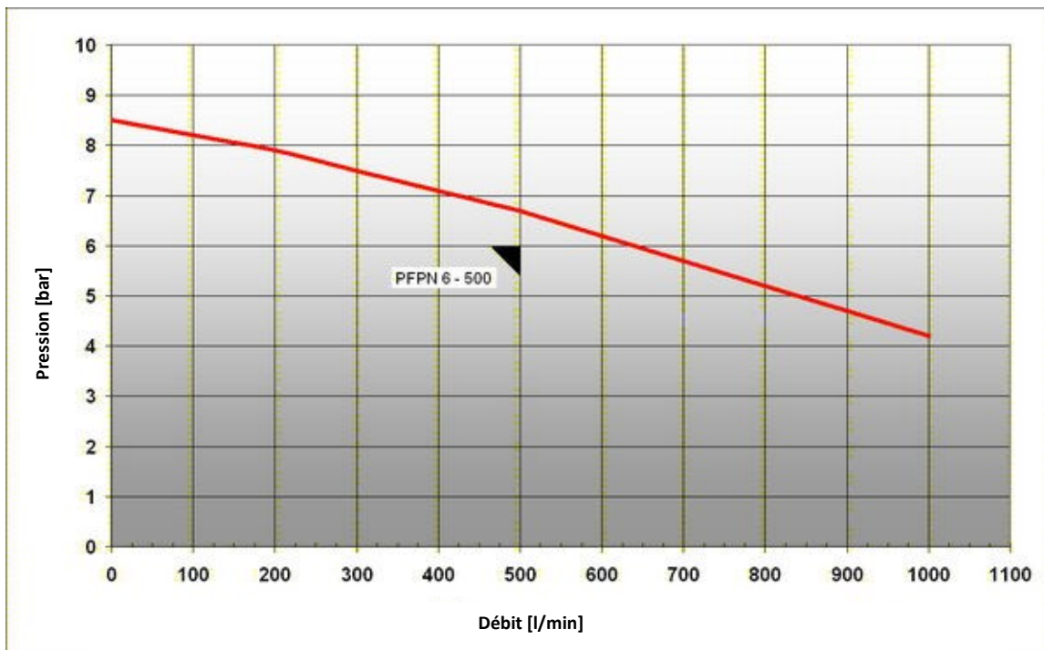
Courbe de puissance
